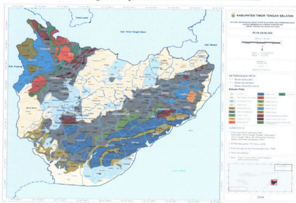
Gambar 2.2 Peta Geologi Kabupaten TTS Menurut Kecamatan
